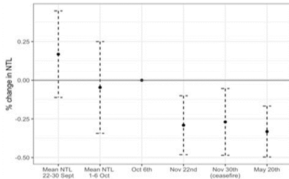
Figure VII Variation en pourcentage de la luminosité nocturne : estimations ponctuelles et intervalles de confiance à 95 %
