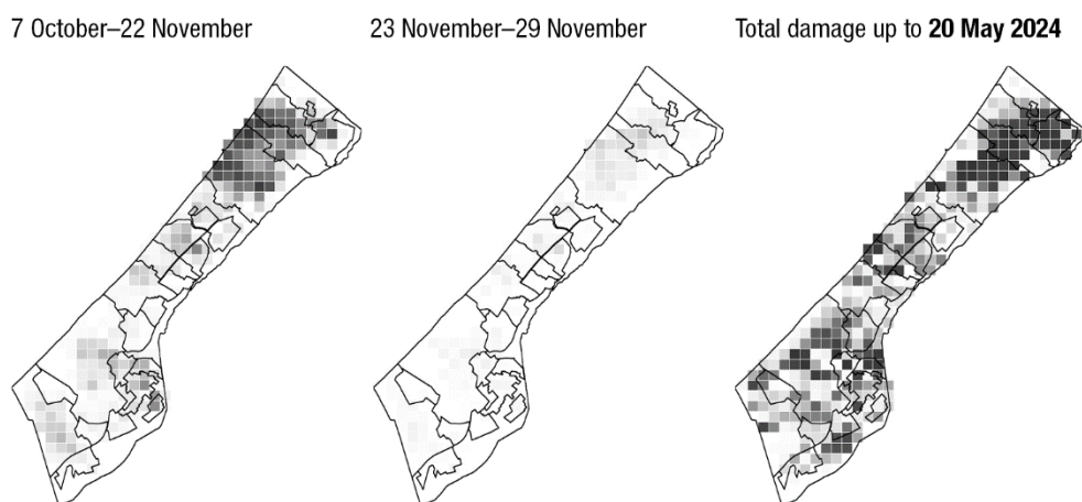
Figure V Intensité des dommages causés au cours de périodes données entre le 7 octobre 2023 et le 20 mai 2024 (mailles de 1 km 2 )
