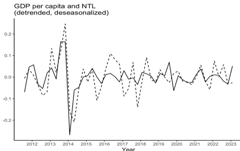
Figure IX Logarithme de la luminosité nocturne et du PIB par habitant, par trimestre (du premier trimestre 2012 au troisième trimestre 2023)
