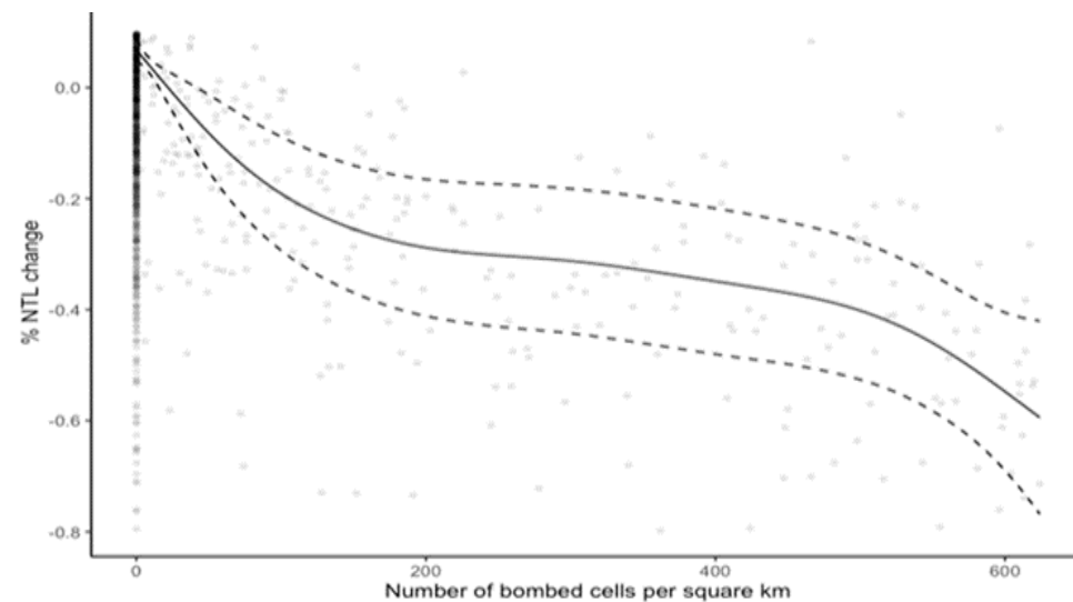
Figure VIII Incidence du nombre de cellules de 40 m x 40 m bombardées par kilomètre carré sur la luminosité nocturne (variation en pourcentage)
