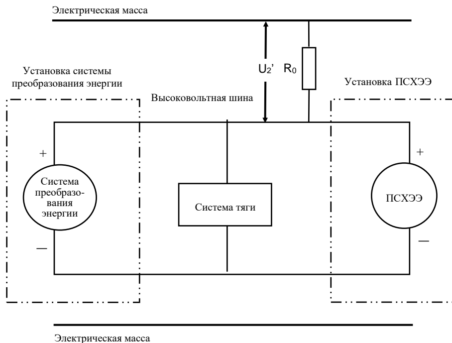
Рис. 6 Измерение U_2'
