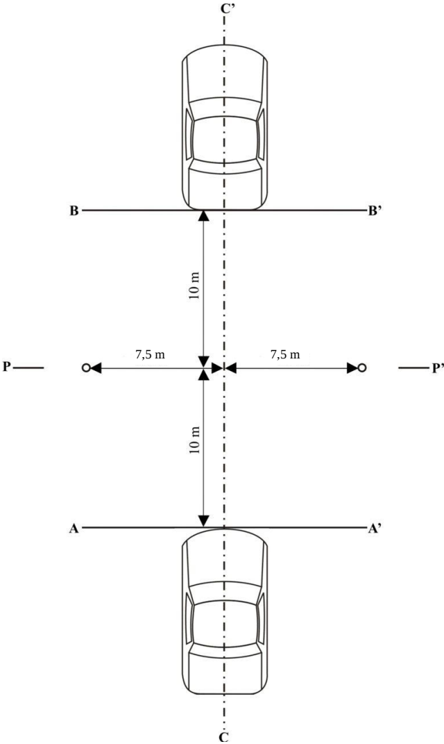
Figure 1 Positions pour l’essai des véhicules en marche
