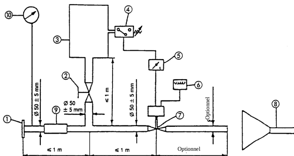
Figure 1 Appareillage de conditionnement
