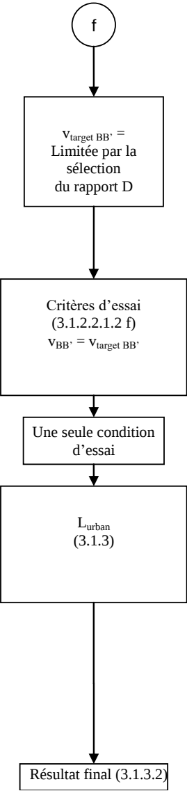
Figure 4c Diagramme de décision pour les véhicules soumis à essai conformément aux dispositions du paragraphe 3.1.2.2 de l'annexe 3 du présent Règlement – Essai rapports non bloqués – 2 e PARTIE
