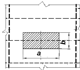
Рис. 10A-2 Площадка нагружения для ребра жесткости
